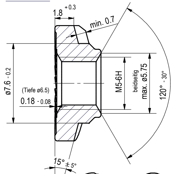
Schnitt A-A
